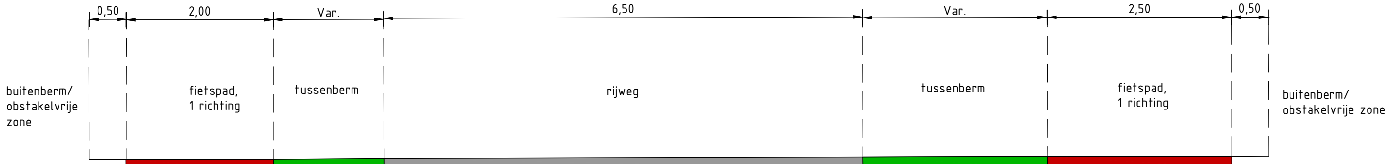
Principeprofiel 4 - deelgebied 03 Principeprofiel - 60 km/uur zone schaal 1:50
